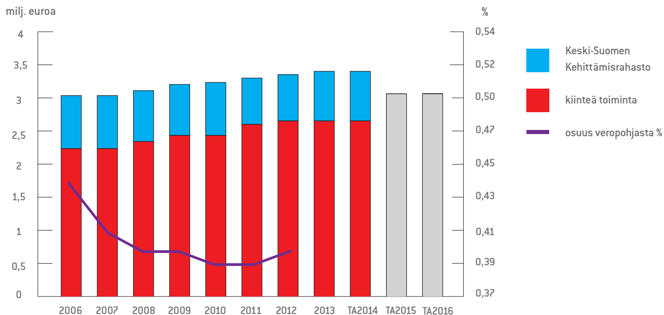
Kuva 4. Kuntien jäsenmaksut (M€) 2006-2016 ja osuus veropohjasta 2006-2012
